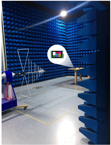
图 4-5 RE 测试图
