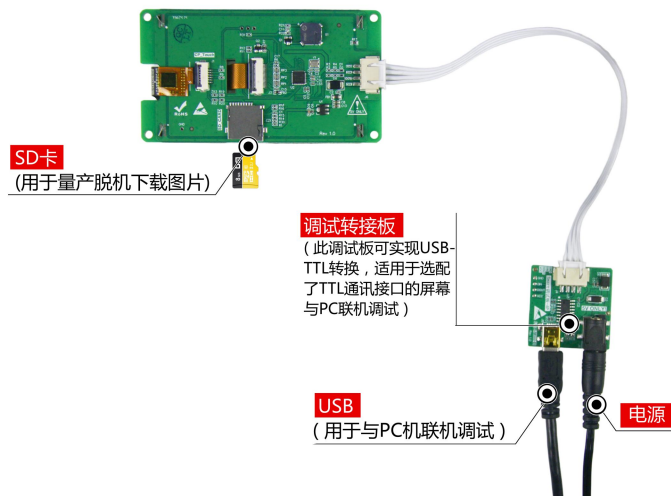
图 1-3 调试工具图
