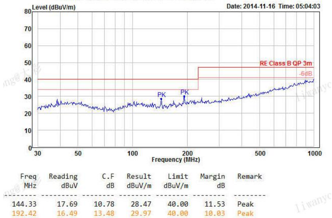
图 4-7 RE 测试垂直方向
