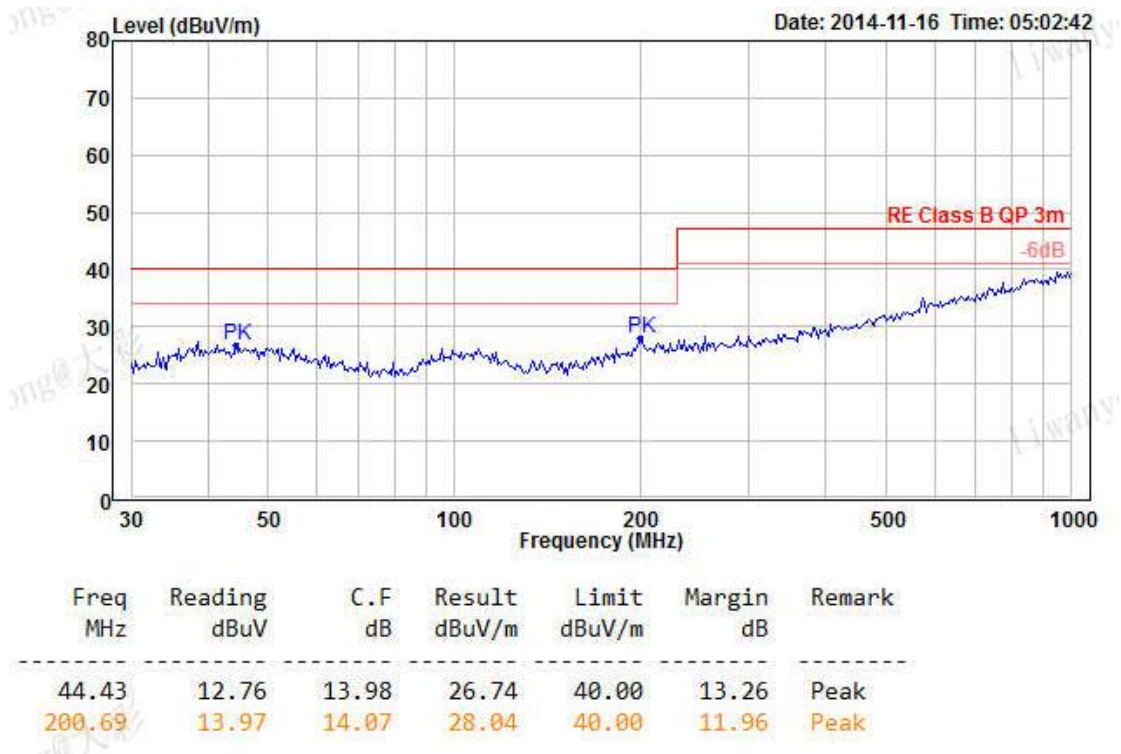
图 4-6 RE 测试水平方向
